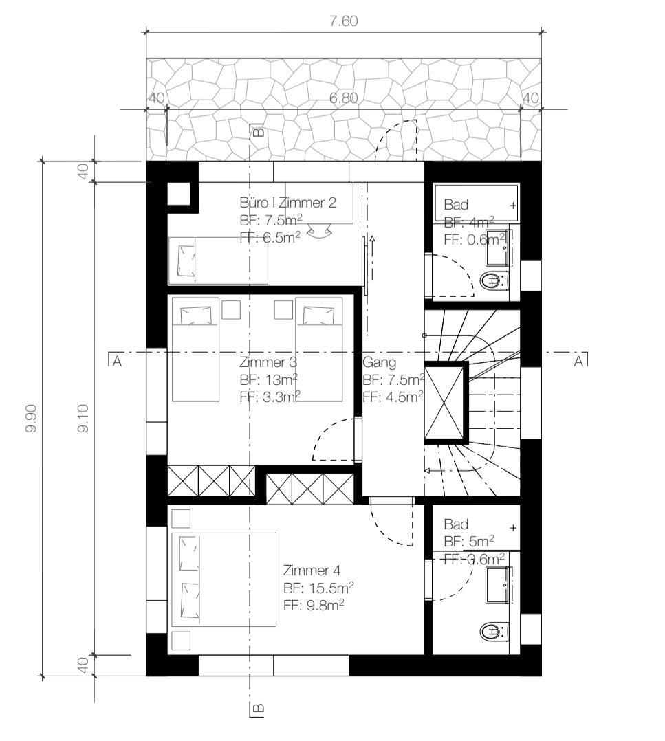
Grundriss OG I 1.100
