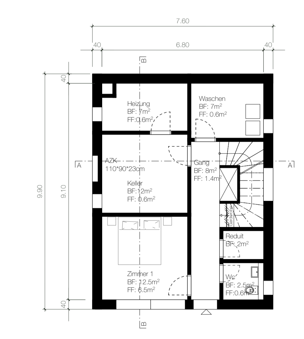
Grundriss EG I 1.100
