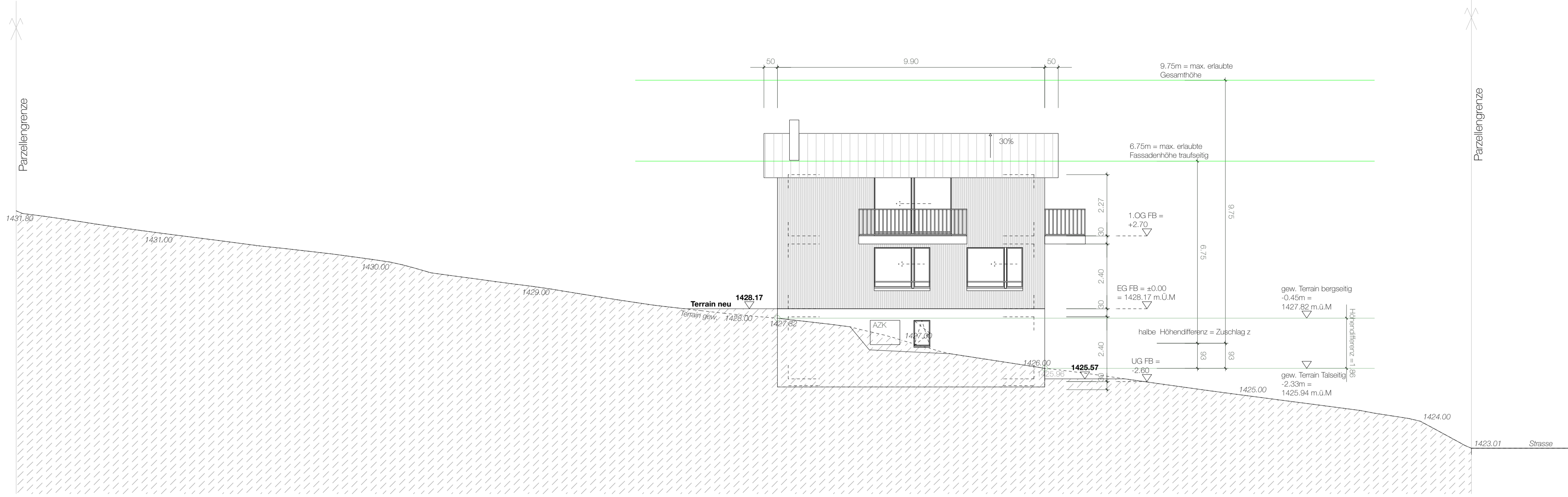
Fassade Süd I 1.100
