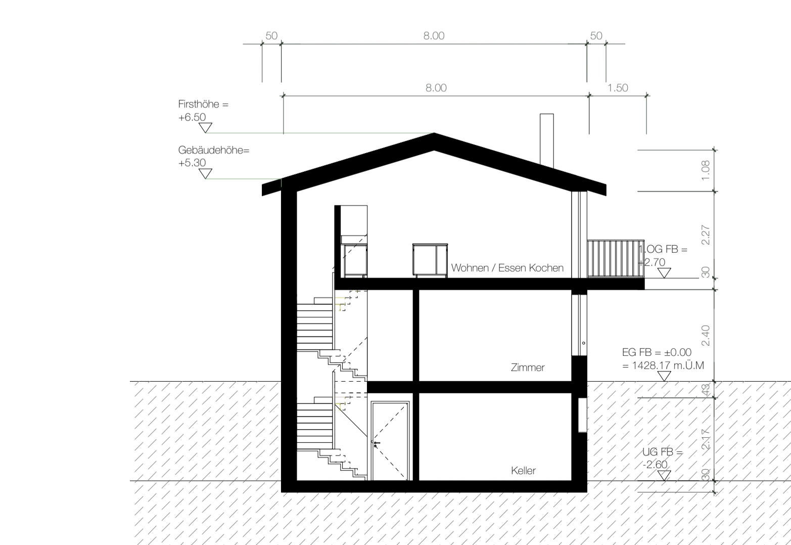
Querschnitt A-A I 1.100
