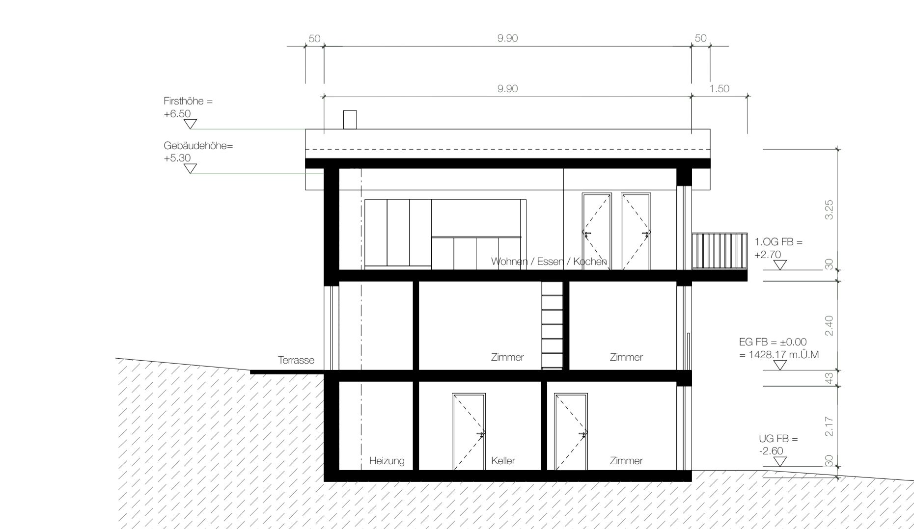
Längsschnitt B-B I 1.100
