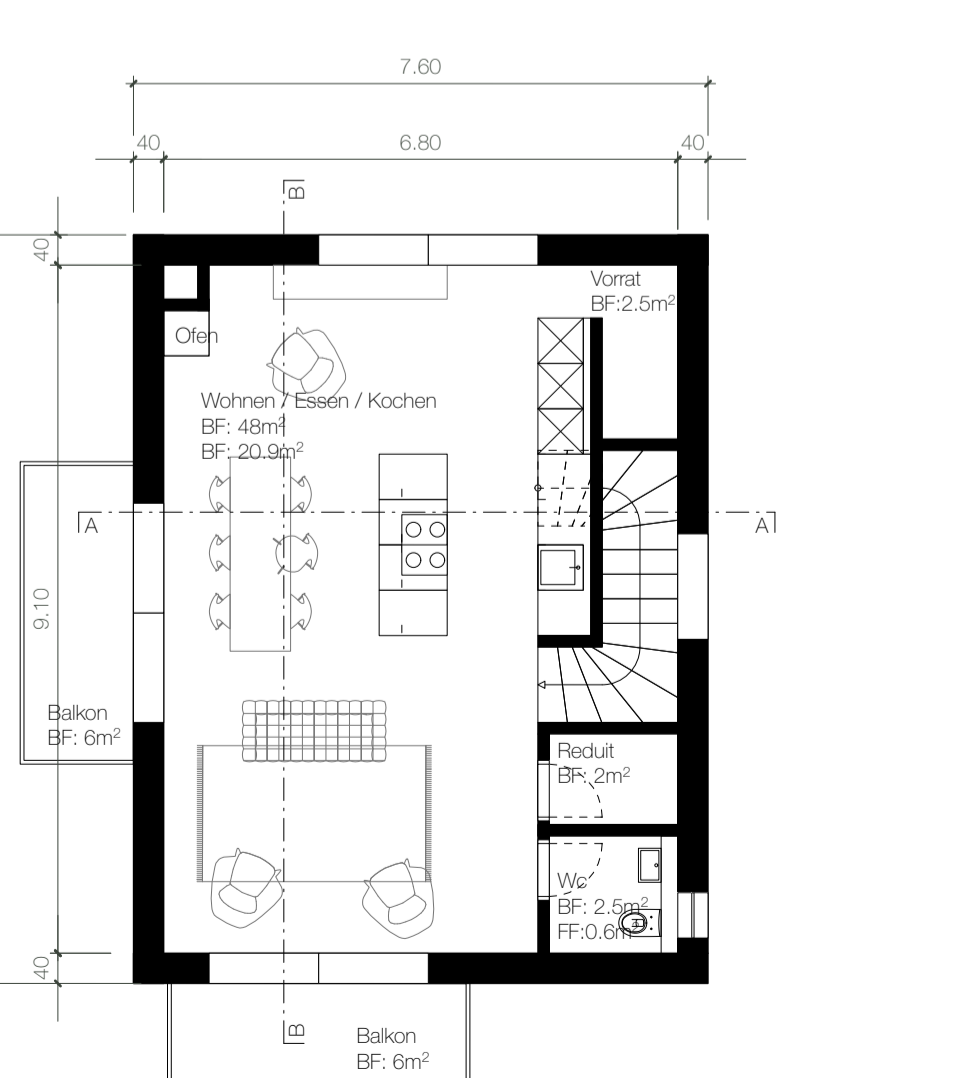
Grundriss DG I 1.100
