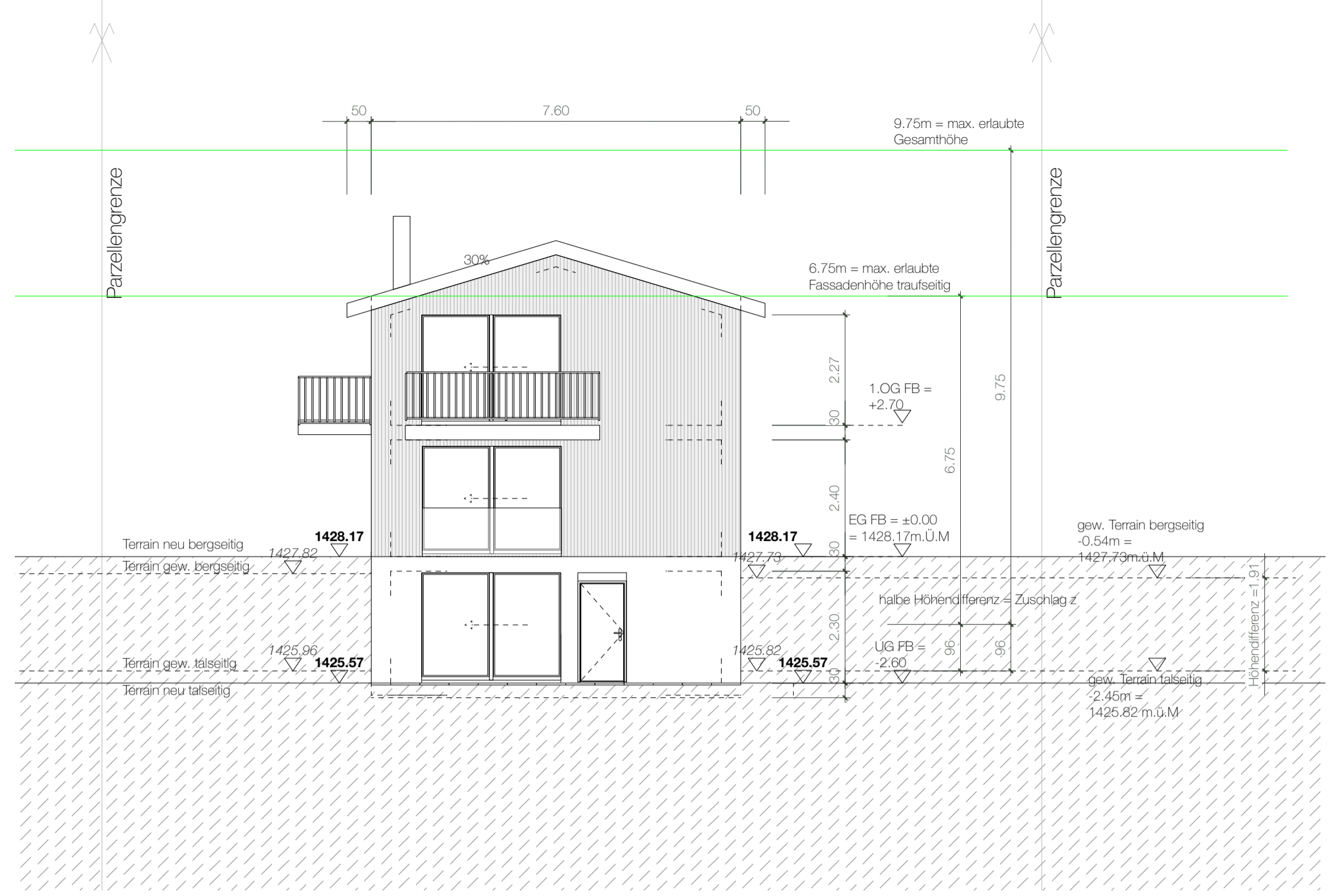
Fassade Ost I 1.100
